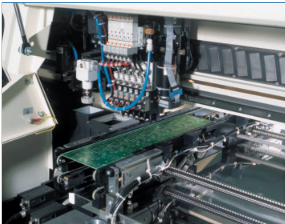
SMD Printed Circuit Board Productielijn.
